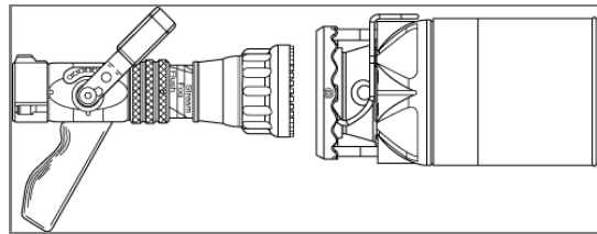
Figure 5.3.1.2.1(d) Multifunction Foam Device.
